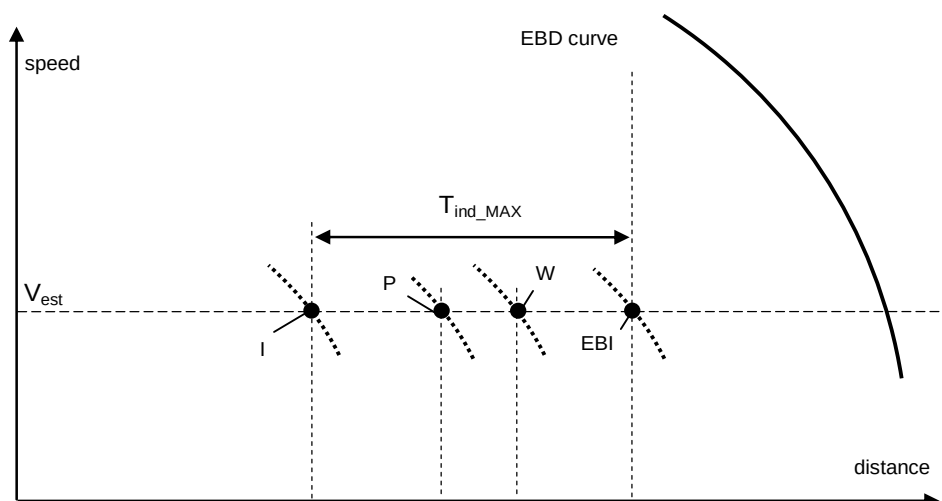
Abbildung 1 – Darstellung der Ankündigungszeit T_{\text{ind\_MAX}}
